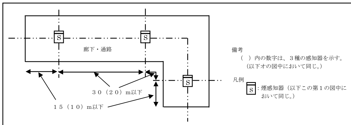
《廊下等における煙感知器の設置例》
