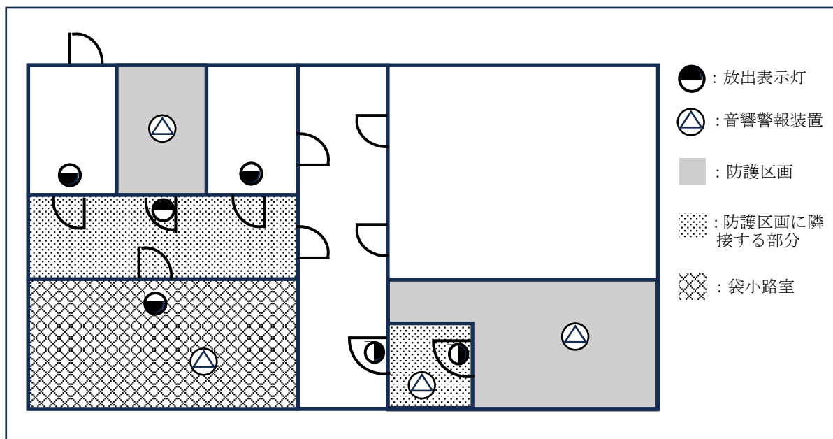
《音響警報装置及び放出表示灯の設置例》
