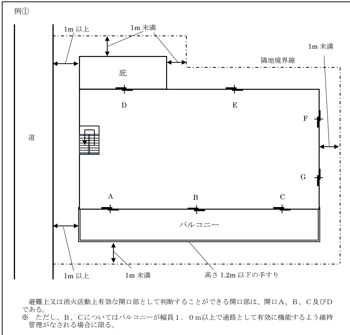
《庇等の設置例2（建築物平面図例）》
