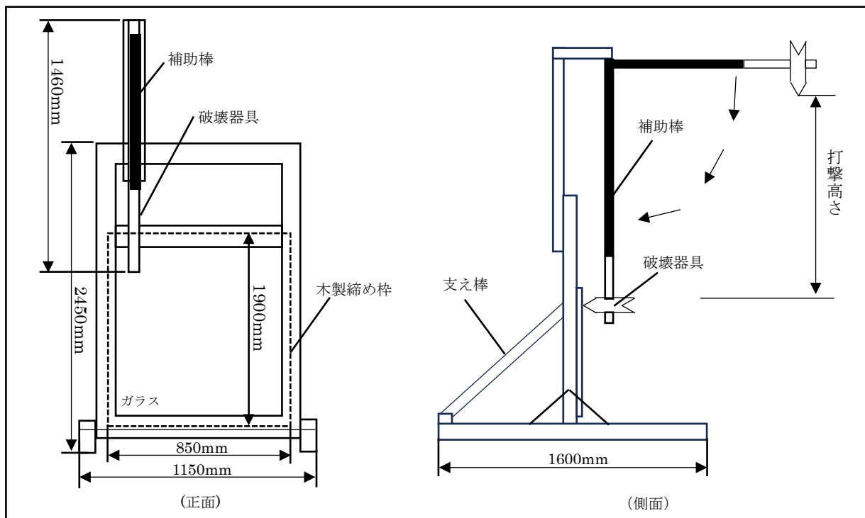
《 図 1 本体 》
