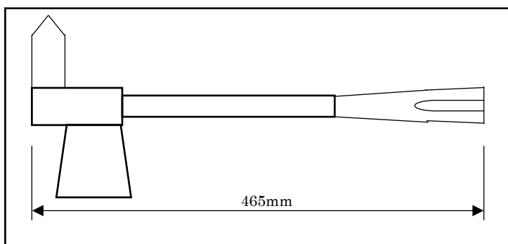
《 図3 破壊器具 》
